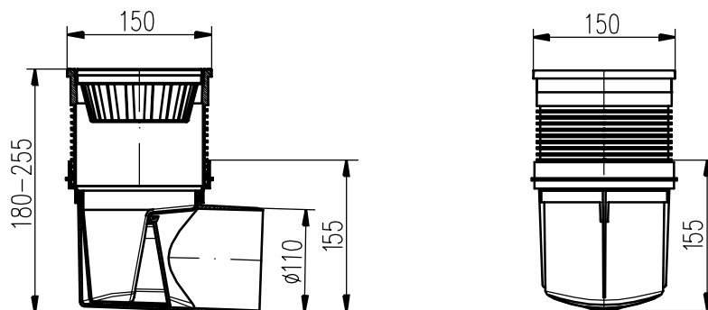
Clapetă anti-miros
